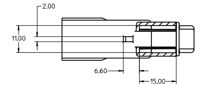
SECTION D-D
